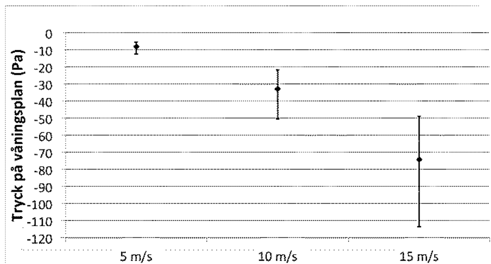
Figur 5: Tryck på våningsplan relativt vindstill för olika vindhastigheter. Viss variation mellan våningar finns, men dessa är små. Ovanstående anger medelvärde för våningarna. Felstaplarna indikerar maximalt respektive minimalt tryck för olika vindriktningar.
