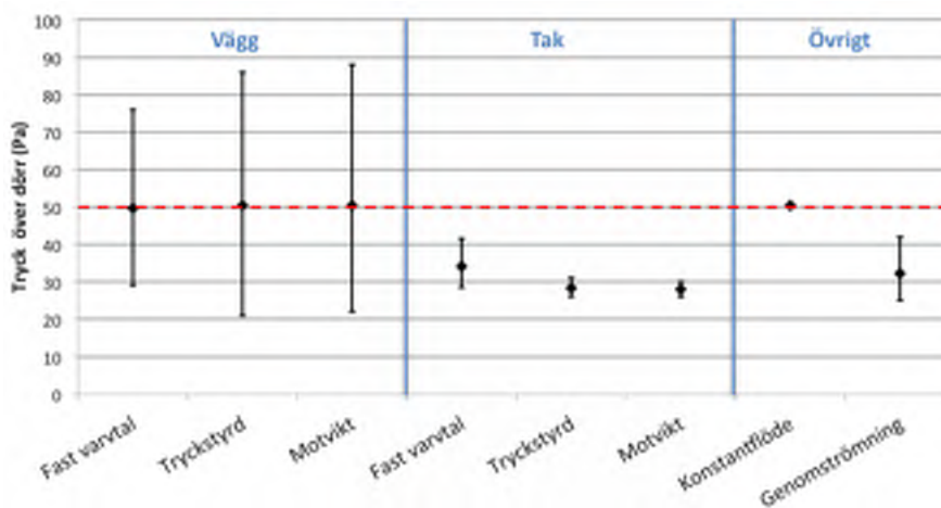
Figur 6: Tryck över dörr vid aktiverat trycksättningsystem för olika systemlösningar vid 5 m/s. Felstaplarna anger variationen beroende på vindriktning relativt byggnaden.
